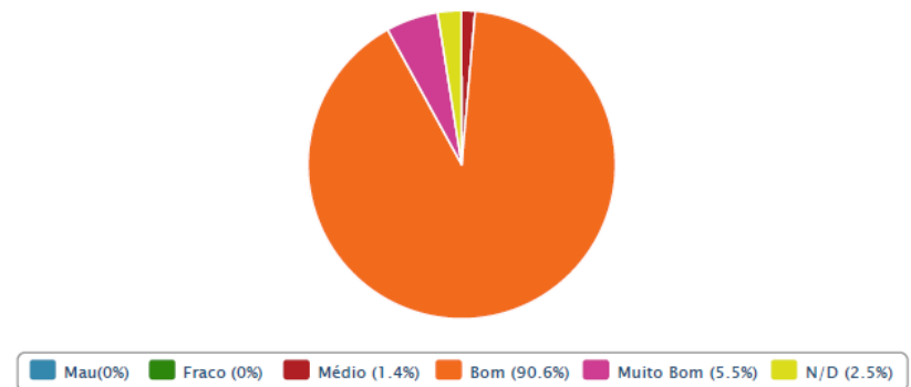
Índice de qualidade do ar da Região obtido para o ozono (O3) em 2013
