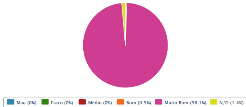
Índice de qualidade do ar da Região obtido para as partículas PM10 em 2013
