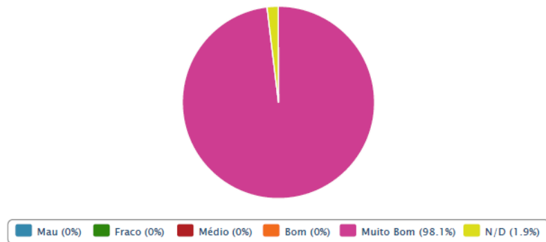
Índice de qualidade do ar da Região obtido para o dióxido de azoto (NO2) em 2013
