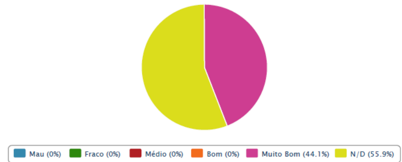
Índice de qualidade do ar da Região obtido para o dióxido de enxofre (SO2) referente a 2013
